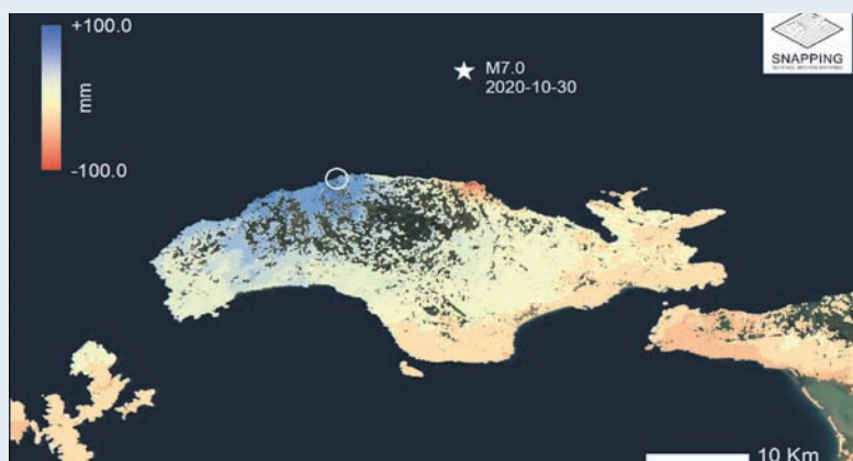
Με το μπλε το τμήμα της Σάμου που ανυψώθηκε κατά δώδεκα εκατοστά και με κόκκινο η περιοχή όπου καταγράφηκε καθίζηση εννέα εκατοστών.
